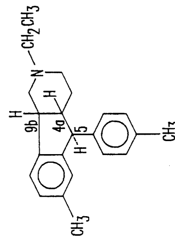
A-4: 4aRS, 5SR, 9bSR 4aβ, 5β, 9bα 4a/9b Trans, 4a/5 Trans
