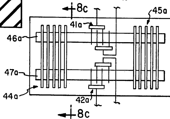
FIG. 8d
