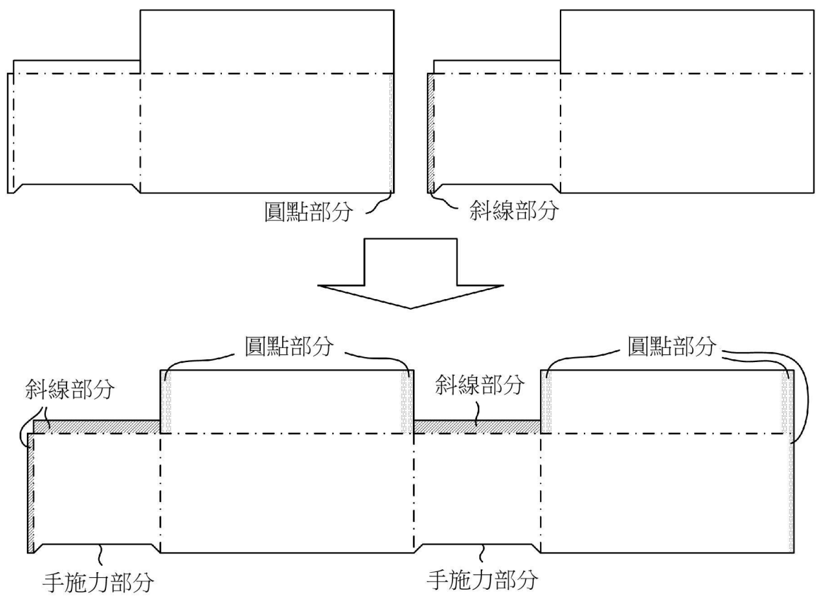
【上箱之參考展開圖】
