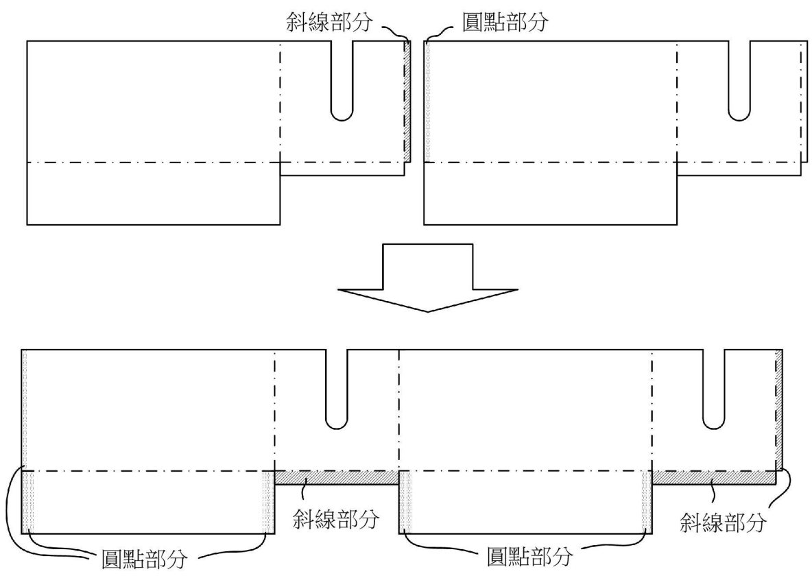
【下箱之參考展開圖】
