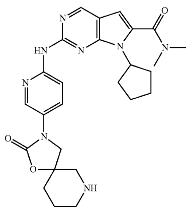
Step 4
