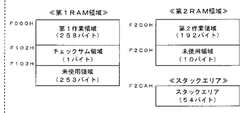
【RAMに係るメモリマップ】
