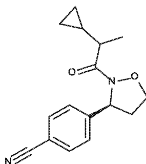
DIASTEREISOISOMER 1
