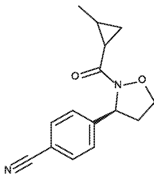
DIASTEREISOMER 2
