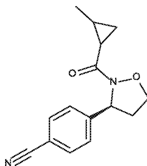
DIASTEREISOMER 1
