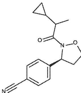
DIASTEREISOISOMER 2
