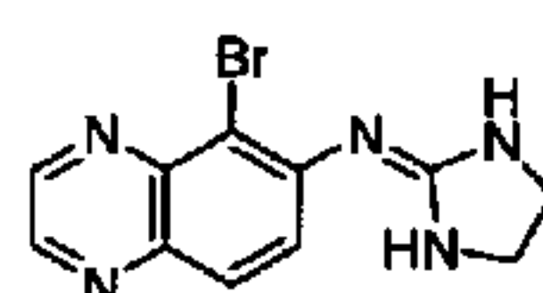
brimonidine
