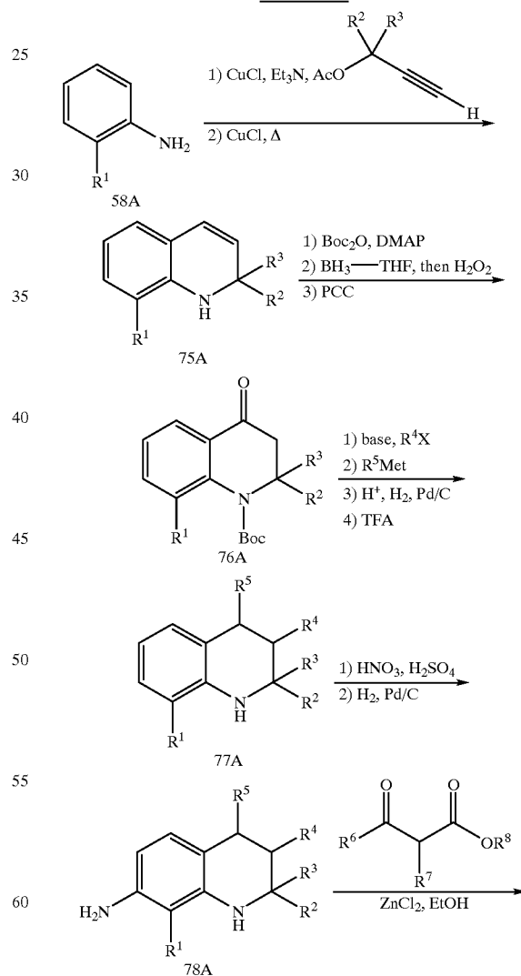
Scheme LIII
