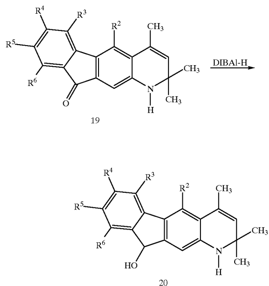
Scheme VI
