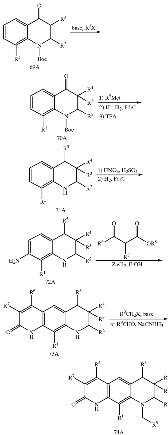
Scheme LII
