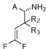
Formula (IVa);
