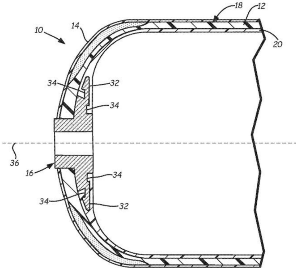
图2 (现有技术)
