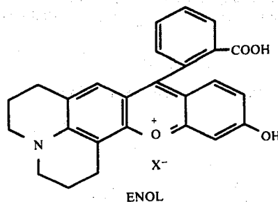
ENOL
