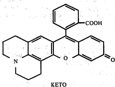
KETO
