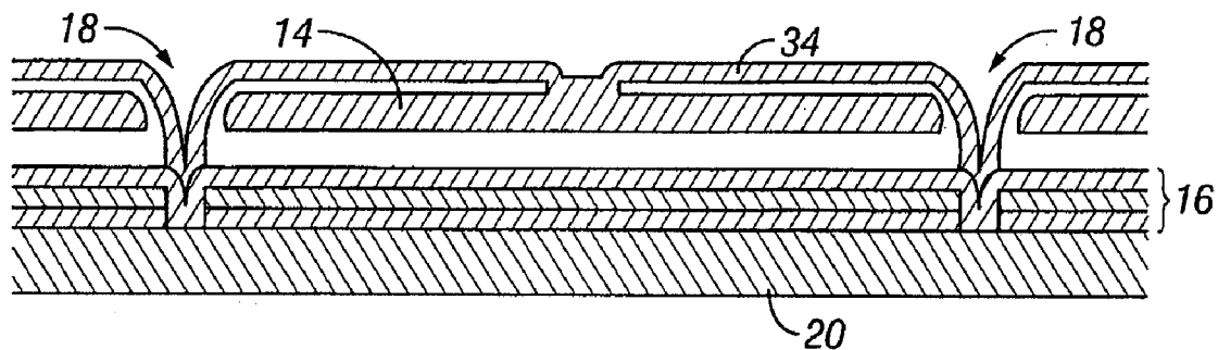
FIG. 7C
