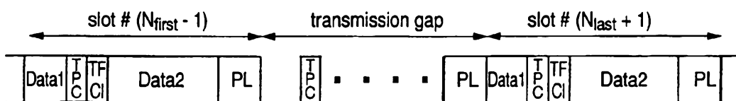
(d) Frame structure type B
