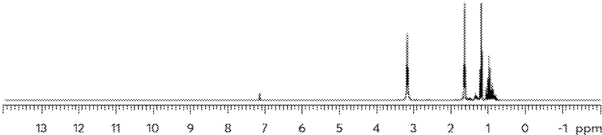
Figure 13: NMR of Et 2 Sn(Pyrolo-dinyl) 2
