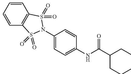
N-(4-(1,1,3,3-tetraoxidobenzo[d][1,3,2]dithiazol-2-yl)phenyl)cyclohexanecarboxamide
