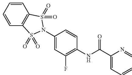
N-(2-fluoro-4-(1,1,3,3-tetraoxidobenzo[d][1,3,2]dithiazol-2-yl)phenyl)picolinamide
