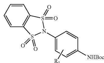
tert-butyl (4-(1,1,3,3-tetraoxido-1,3,2-dithiazol-2-yl)phenyl)carbamate
