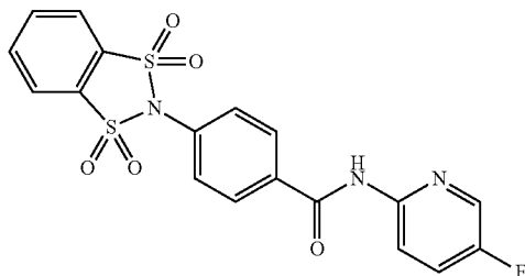
N-(5-fluoropyridin-2-yl)-4-(1,1,3,3-tetraoxidobenzo[d][1,3,2]dithiazol-2-yl)benzamide
