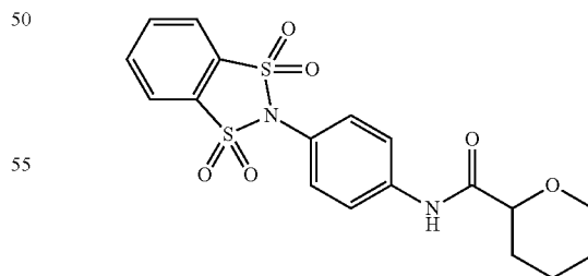
N-(4-(1,1,3,3-tetraoxidobenzo[d][1,3,2]dithiazol-2-yl)phenyl)tetrahydro-2H-pyran-2-carboxamide
