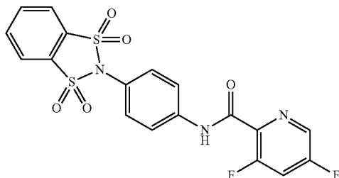
3,5-Difluoro-N-(4-(1,1,3,3-tetraoxidobenzo[d][1,3,2]dithiazol-2-yl)phenyl)picolinamide
