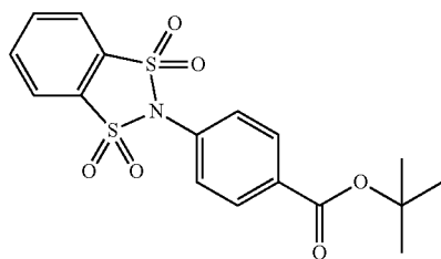
tert-butyl-4-(1,1,3,3-tetraoxido-4-(pyridin-2-yl)-1,3-dithiazol-2-yl)benzoate
