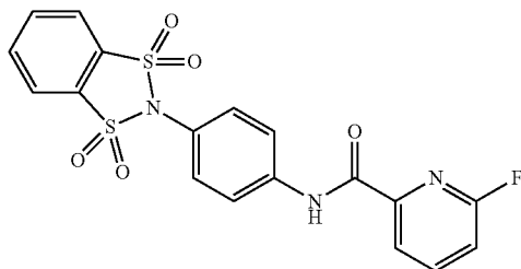
6-Fluoro-N-(4-(1,1,3,3-tetraoxidobenzo[d][1,3,2]dithiazol-2-yl)phenyl)picolinamide
