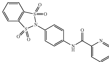
N-(4-(1,1,3,3-tetraoxidobenzo[d][1,3,2]dithiazol-2-yl)phenyl)picolinamide
