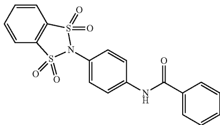
N-(4-(1,1,3,3-tetraoxidobenzo[d][1,3,2]dithiazol-2-yl)phenyl)benzamide
