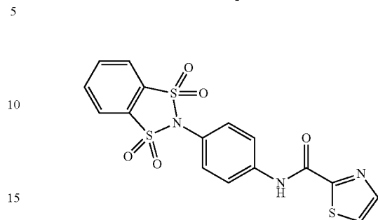
N-(4-(1,1,3,3-tetraoxidobenzo[d][1,3,2]dithiazol-2-yl)phenyl)thiazole-2-carboxamide
