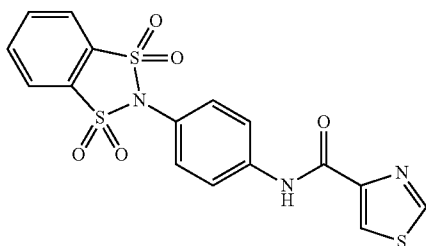
N-(4-(1,1,3,3-tetraoxidobenzo[d][1,3,2]dithiazol-2-yl)phenyl)thiazole-4-carboxamide
