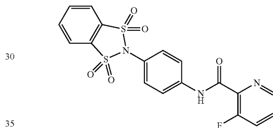
3-Fluoro-N-(4-(1,1,3,3-tetraoxidobenzo[d][1,3,2]dithiazol-2-yl)phenyl)picolinamide
