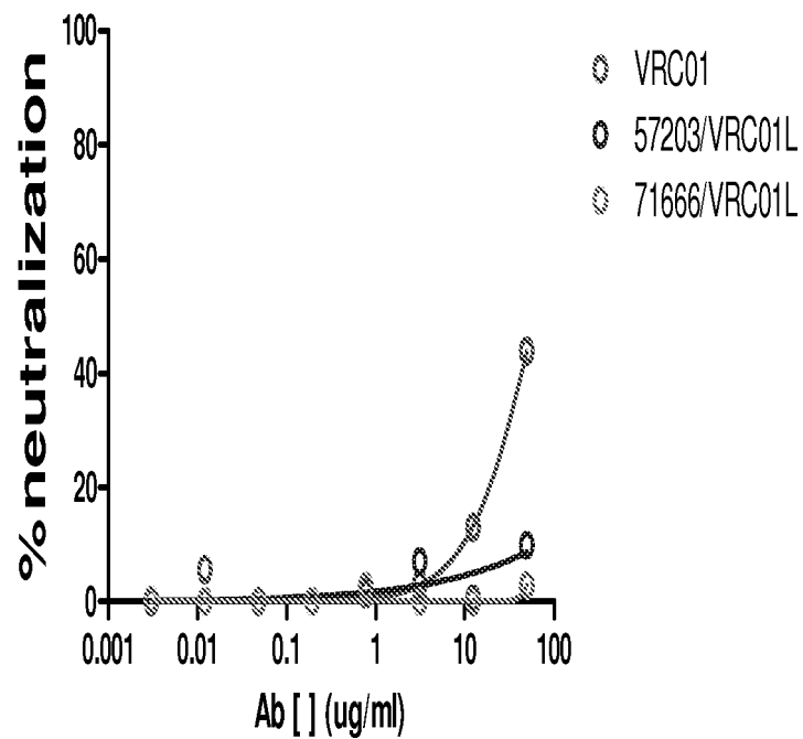
FIG. 81H SIVmac251.30.SIV
