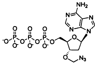
3'-O-Azido-dATP
