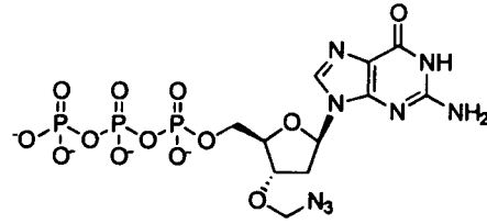
3'-O-Azido-dGTP
