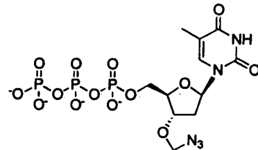
3'-O-Azido-dTTP
