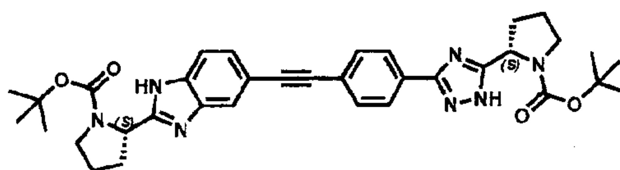
Example 1-441.
