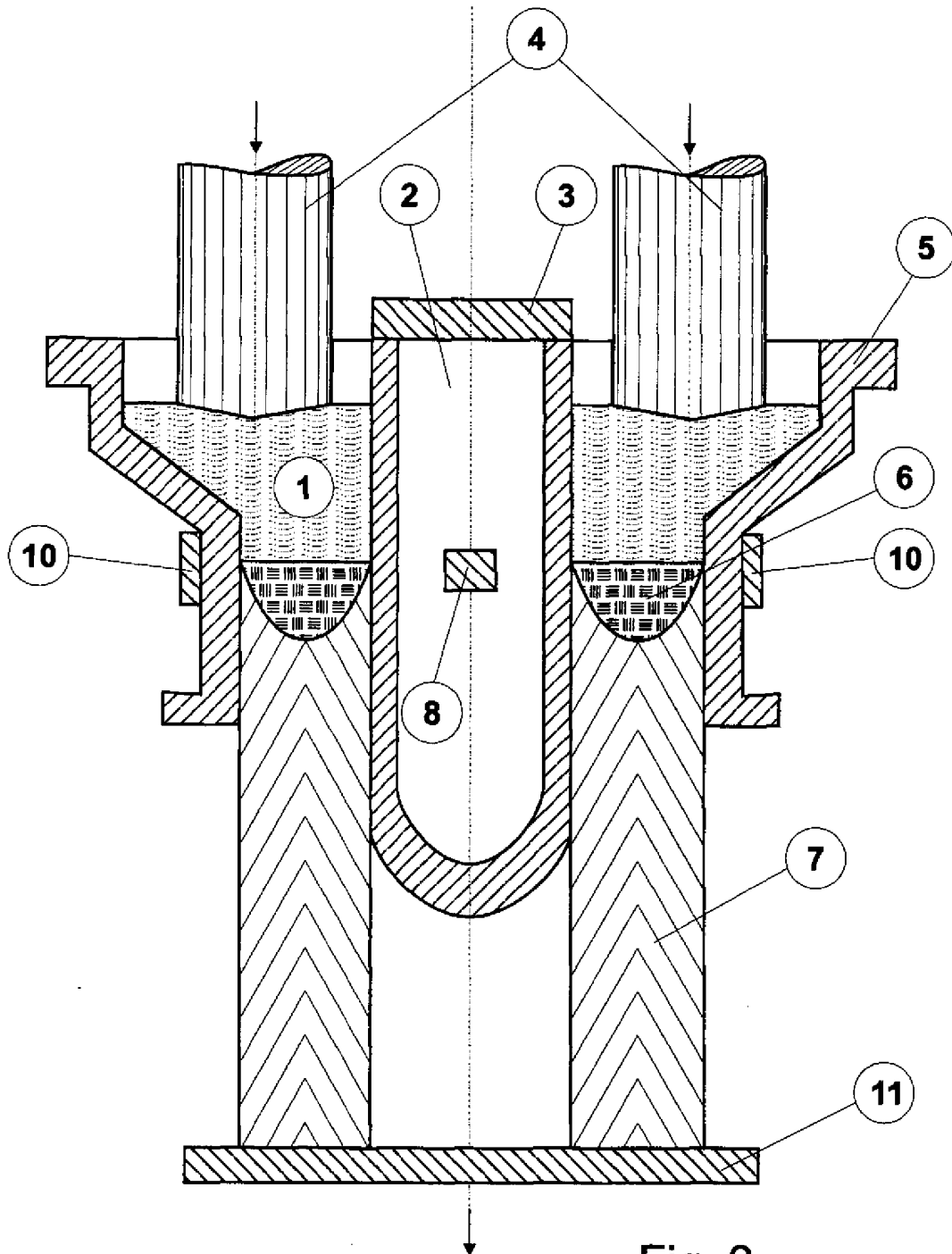
Fig. 2 Schnitt A-A
