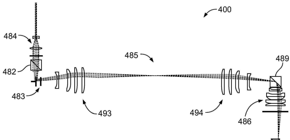
레이저/SLD 빔 전달 광학기기
