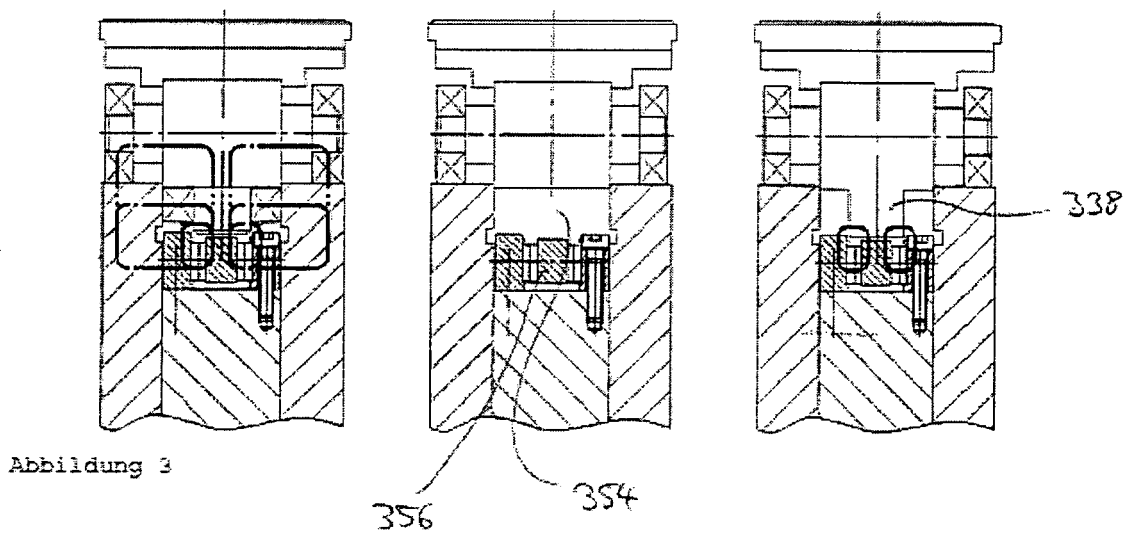
Schnitt A-A Schnitt B-B ohne Steg Schnitt B-B mit Steg Abb. 3.4 Abb. 3.5 Abb. 3.6
