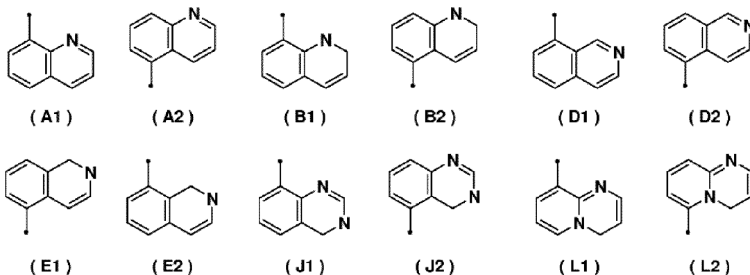
[Chemische Formel 17]
