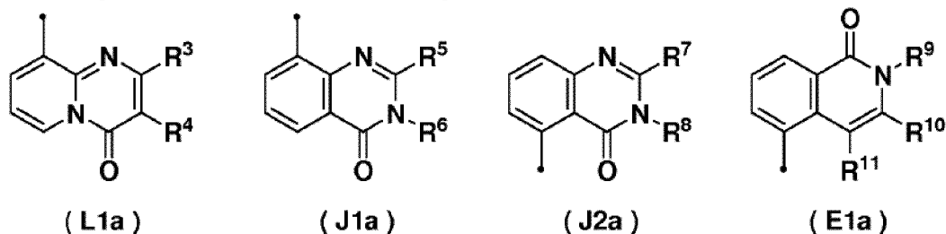
[Chemische Formel 18]
