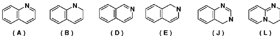
[Chemische Formel 15]
