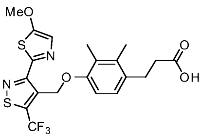
, Cpd 268
