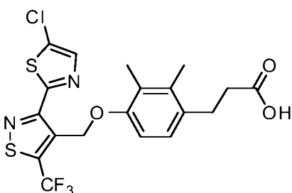
, Cpd 269
