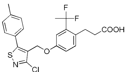
Cpd 278
