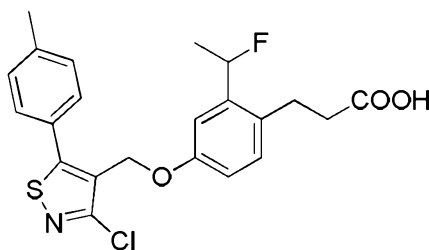
Cpd 279
