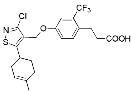
Cpd 276
