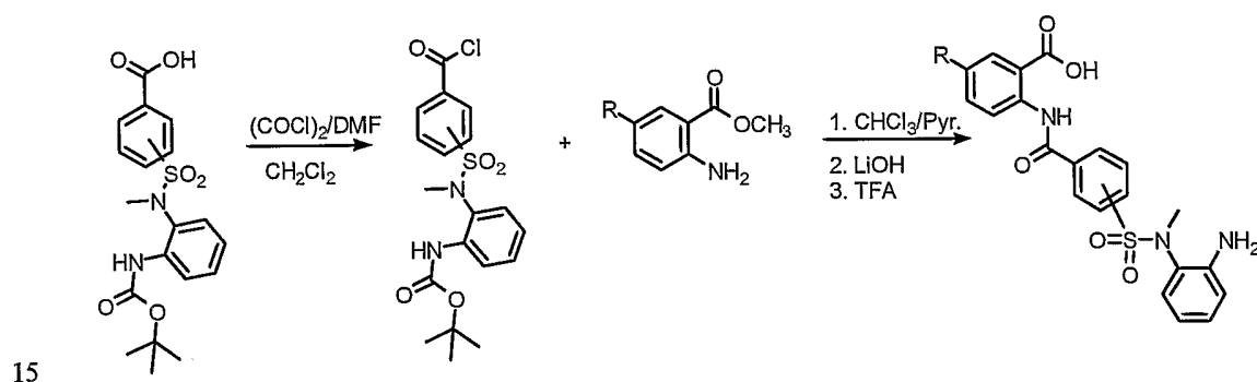
Scheme 1.4
