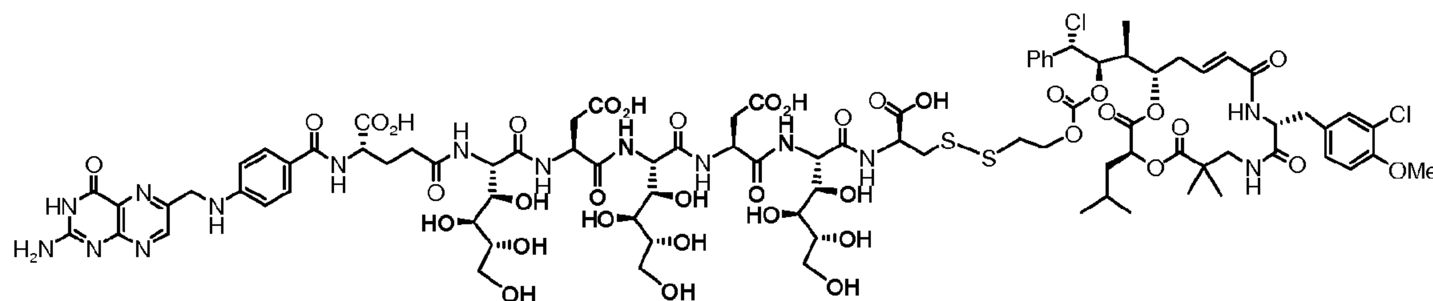
EC0262 Cryptophycin-Carbonate-CH 2 CH 2 -SS-Cys-Saccharo-Asp-Saccharo-Asp-Saccharo-
