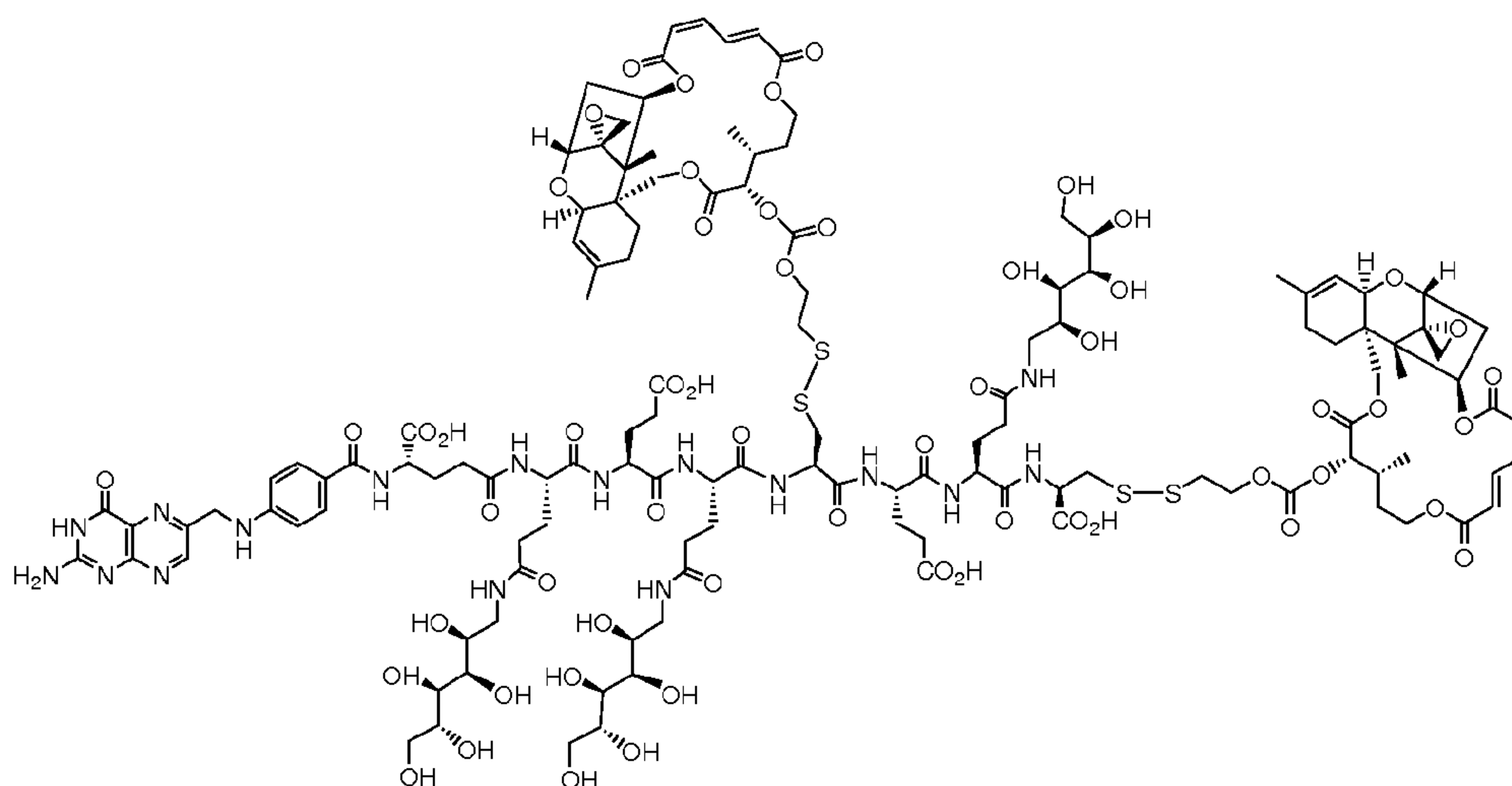
EC0605 Bis-verucaric conjugate.
