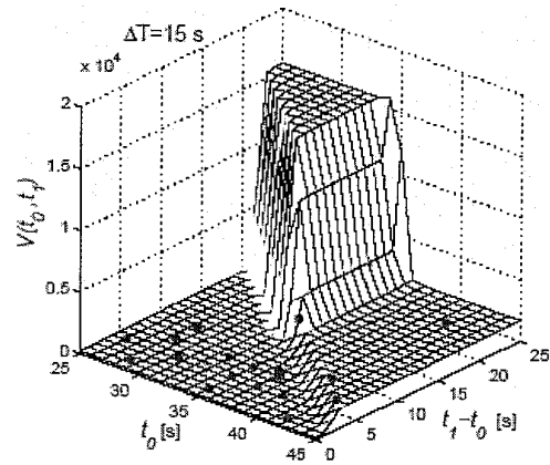
(b) t_0=37.6s ; t_f-t_0=9,2s ; n= 28
