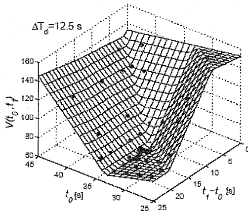
(a) t_0=34.8s ; t_f-t_0=12,5s ; n= 42
