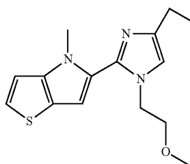
102 5-[4-ethyl-1-(2-methoxyethyl)imidazol-2-yl]-4-methyl-thieno[3,2-b]pyrrole
