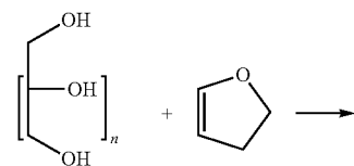
Scheme 28.
