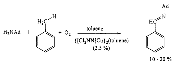
Scheme 30.
