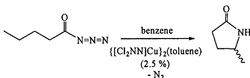
Scheme 19.
