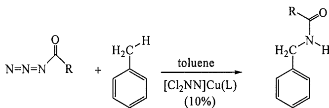
Scheme 25.
