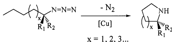
Scheme 20.
