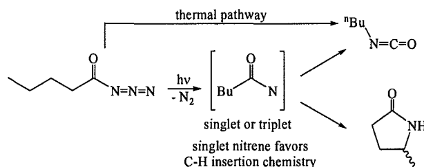
Scheme 16.
