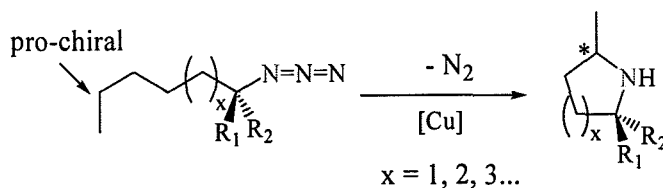
Scheme 21.
