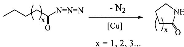
Scheme 26.
