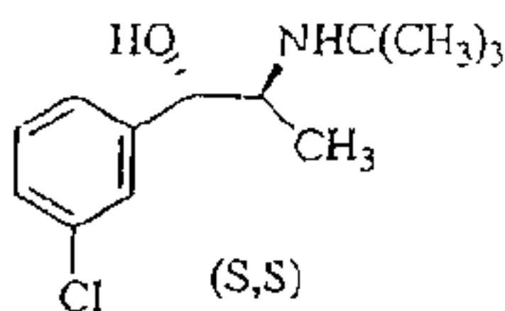
(S,S)-2-(tert-Butylamino)-1-(3-chlorophenyl)-propan-1-ol
