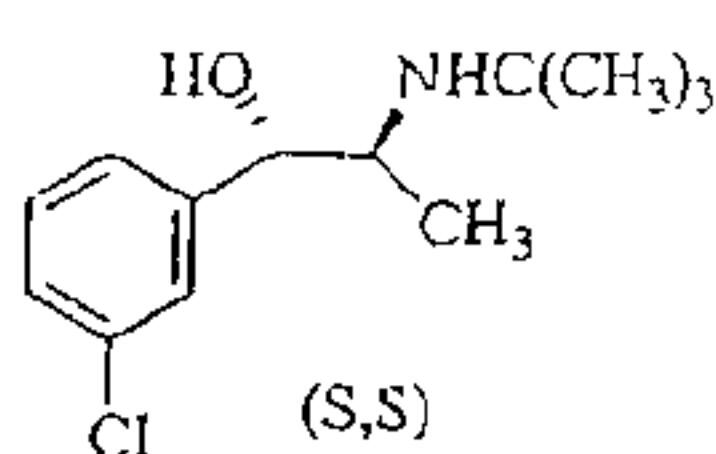
(S,S)-2-(tert-Butylamino)-1-(3-chlorophenyl)-propan-1-ol
