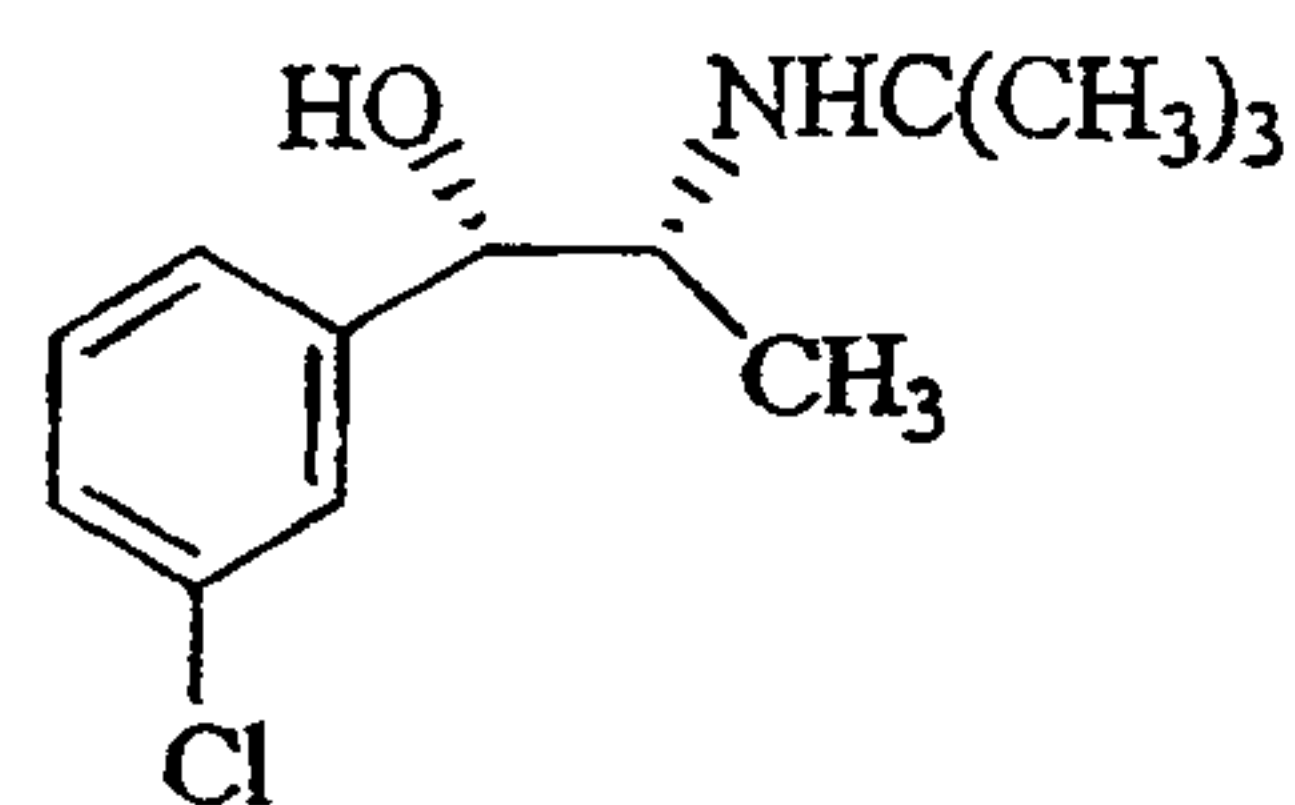
(S,R)-2-(tert-Butylamino)-1-(3-chlorophenyl)-propan-1-ol
