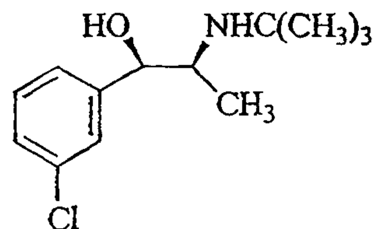
(R,S)-2-(tert-Butylamino)-1-(3-chlorophenyl)-propan-1-ol
