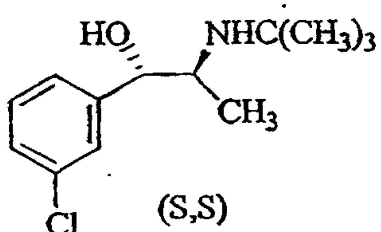
(S,S)-2-(tert-Butylamino)-1-(3-chlorophenyl)-propan-1-ol
