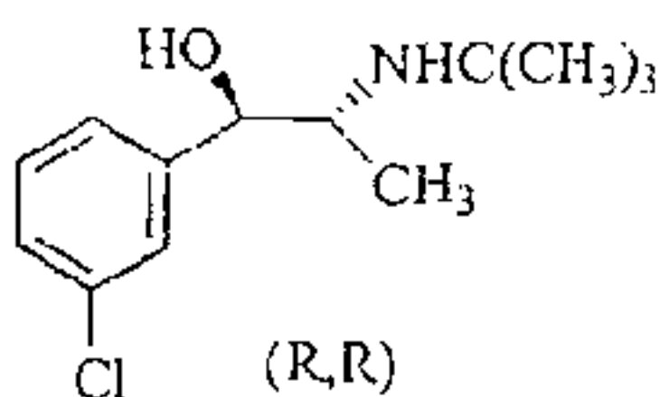
(R,R)-2-(tert-Butylamino)-1-(3-chlorophenyl)-propan-1-ol
