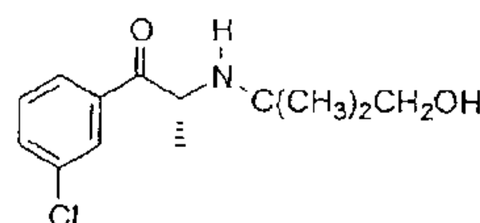
(R)-1-(3-Chlorophenyl)-2-[(1,1-dimethylethanol)amino]-1-propanone
