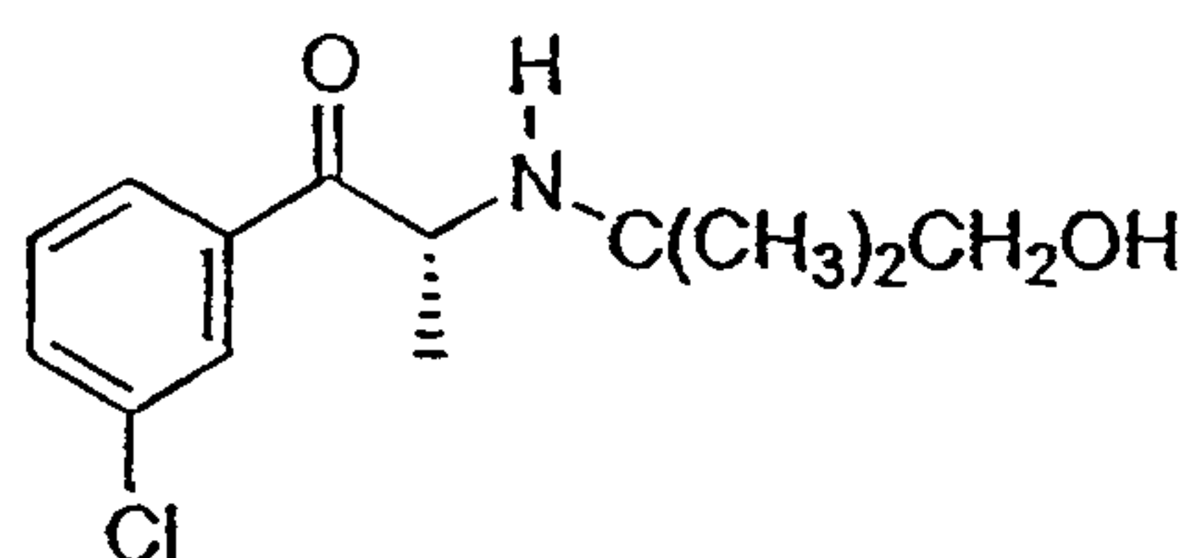
(R)-1-(3-Chlorophenyl)-2-[(1,1-dimethylethanol)amino]-1-propanone
