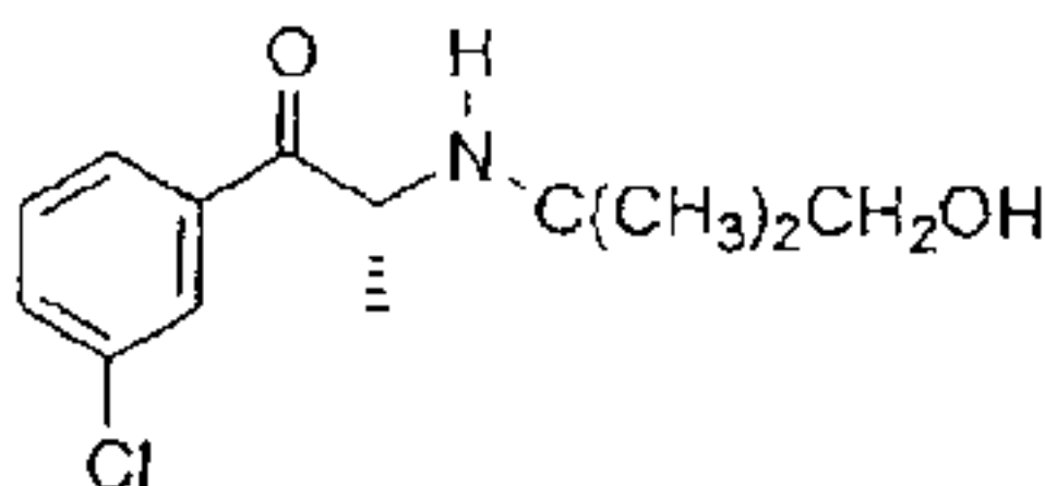
(R)-1-(3-Chlorophenyl)-2-[(1,1-dimethylethanol)amino]-1-propanone
