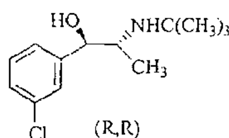
(R,R)-2-(tert-Butylamino)-1-(3-chlorophenyl)-propan-1-ol
