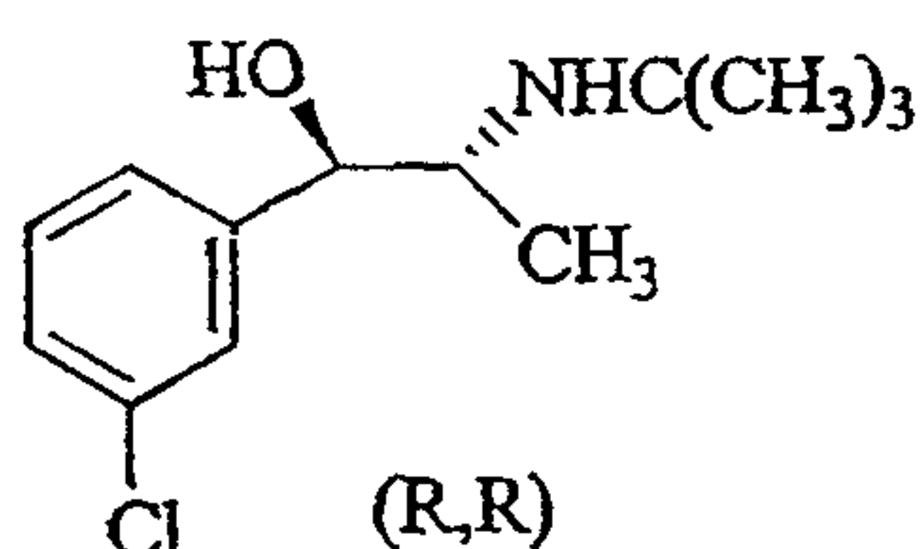
(R,R)-2-(tert-Butylamino)-1-(3-chlorophenyl)-propan-1-ol
