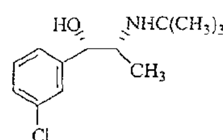
(S,R)-2-(tert-Butylamino)-1-(3-chlorophenyl)-propan-1-ol
