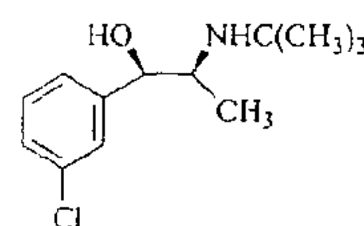
(R,S)-2-(tert-Butylamino)-1-(3-chlorophenyl)-propan-1-ol
