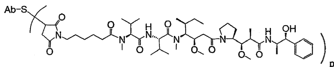
Ab-MC-MMAE
