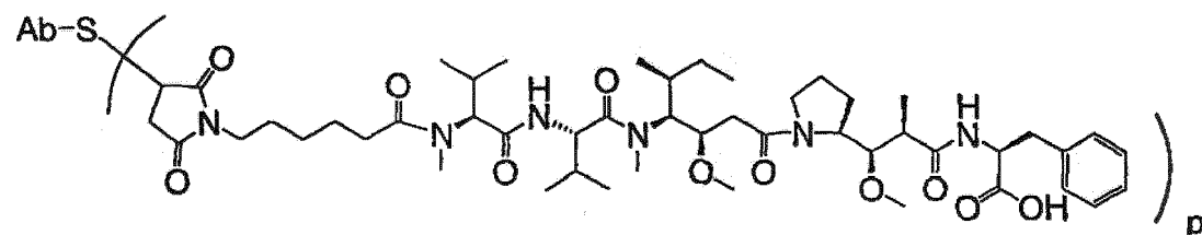
Ab-MC-MMAF
