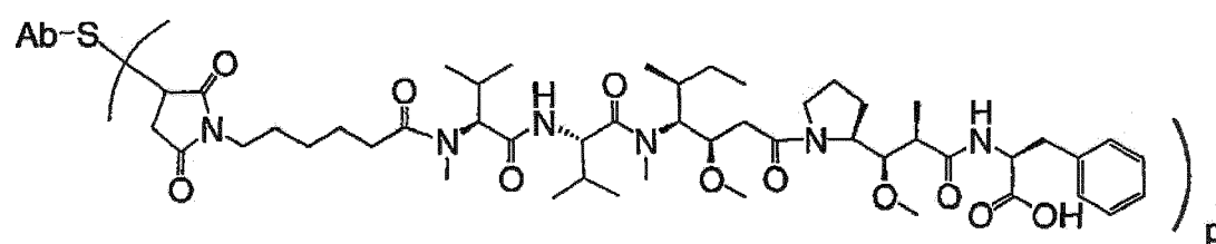
Ab-MC-MMAF
