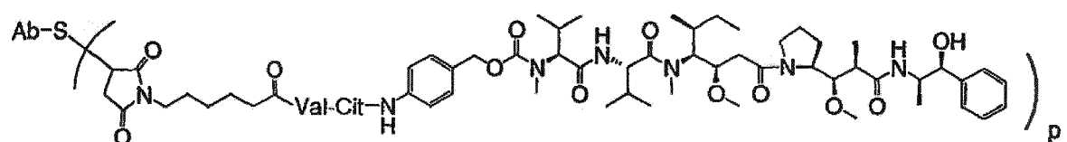
Ab-MC-vc-PAB-MMAE
