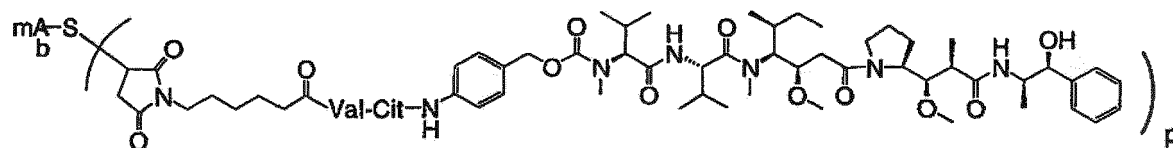
L-MC-vc-PAB-MMAE
