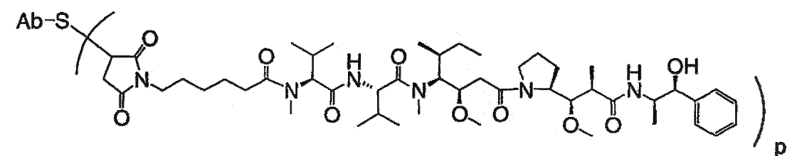
Ab-MC-MMAE
