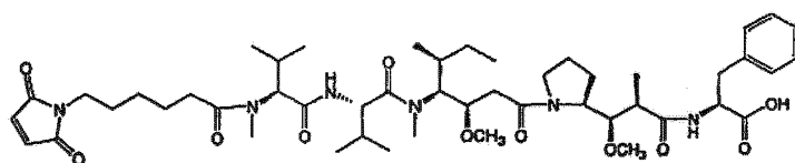
MC-MMAF
