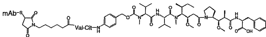
L-MC-vc-PAB-MMAF
