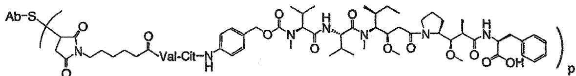
Ab-MC-vc-PAB-MMAF
