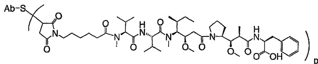
Ab-MC-MMAF
