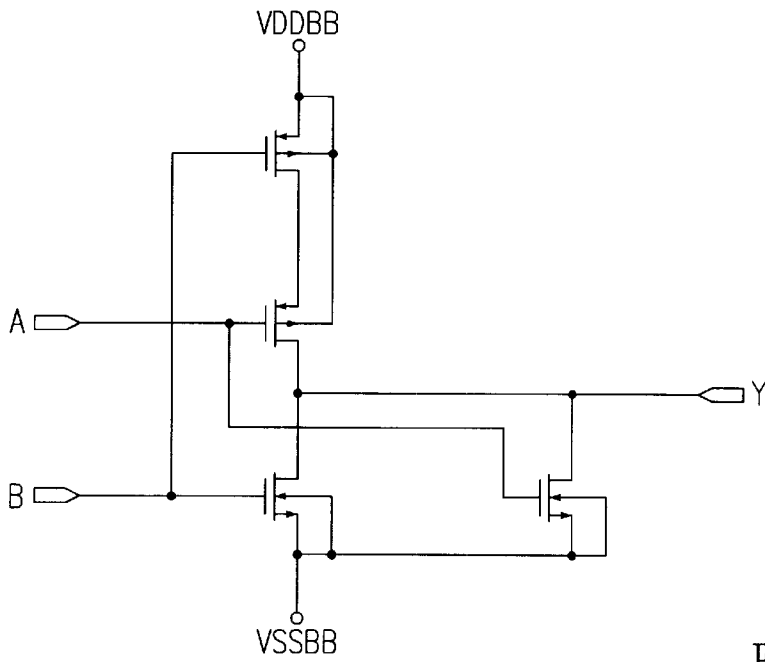
NOR2
