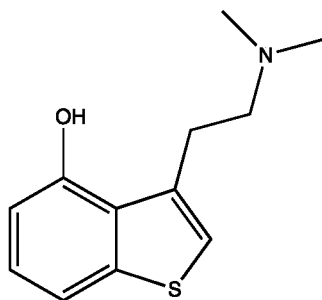
Thiopsil™
