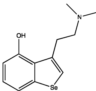
Selenopsil™
