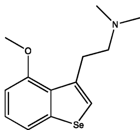
4-methoxy Selenopsil™
