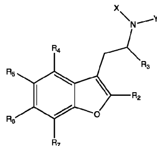
Formula Ic
