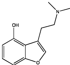
Furanopsil™
