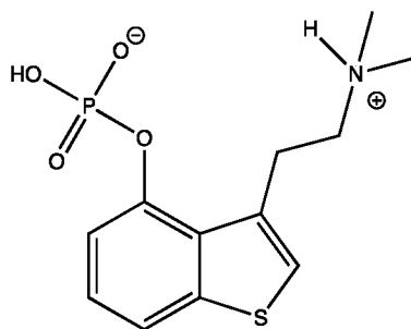
Thiocybin™
