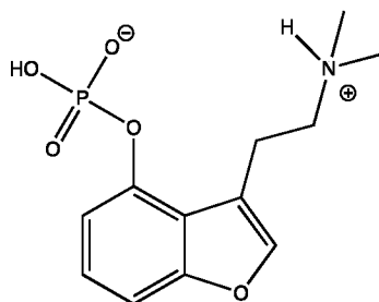
Furocybin™
