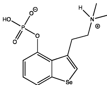
Selenocybin™
