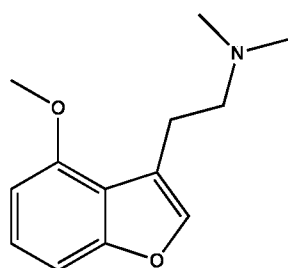
4-methoxy Furanopsil™
