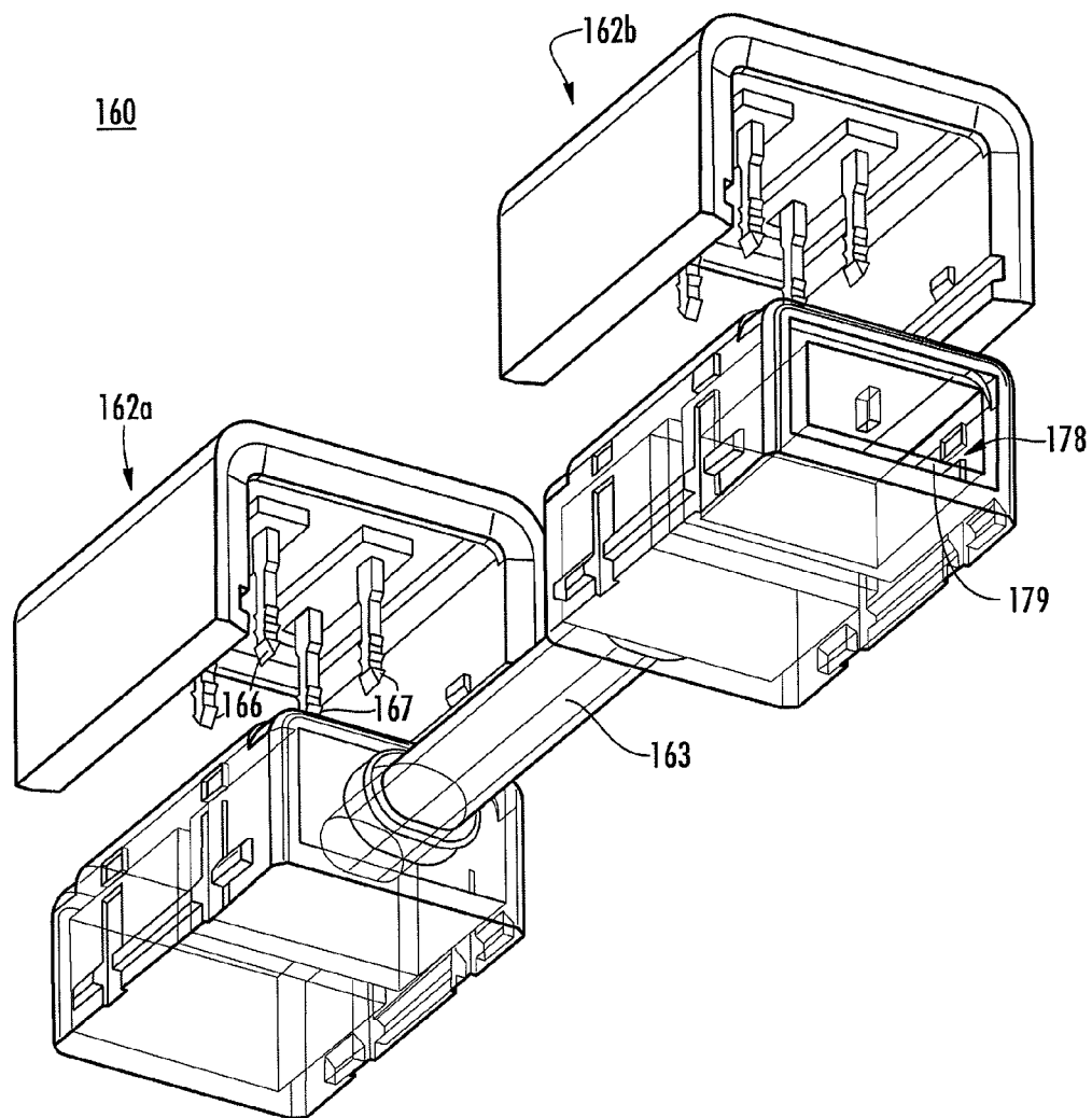
FIG. 30A
