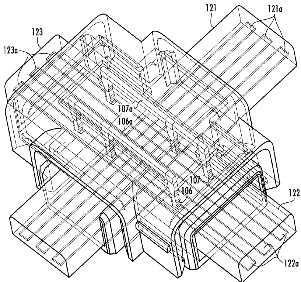
FIG. 23A
