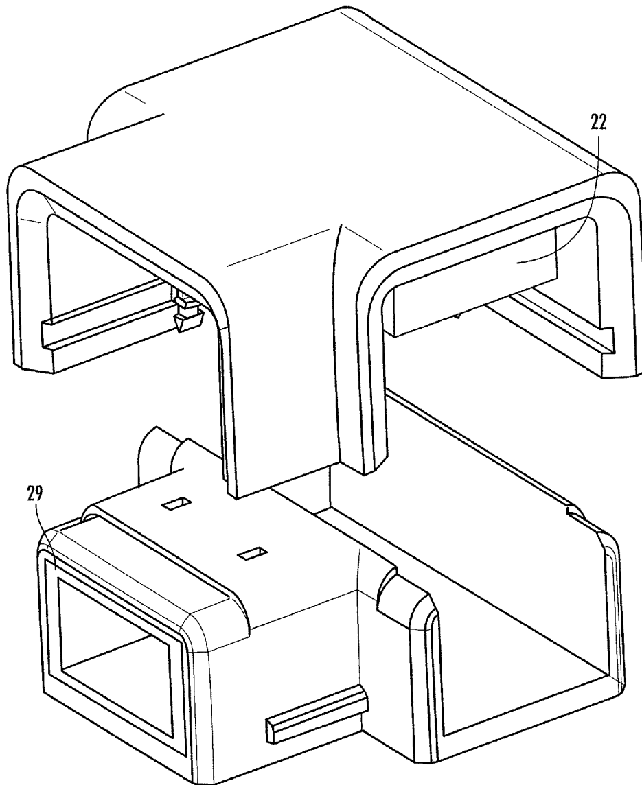
FIG. 5B
