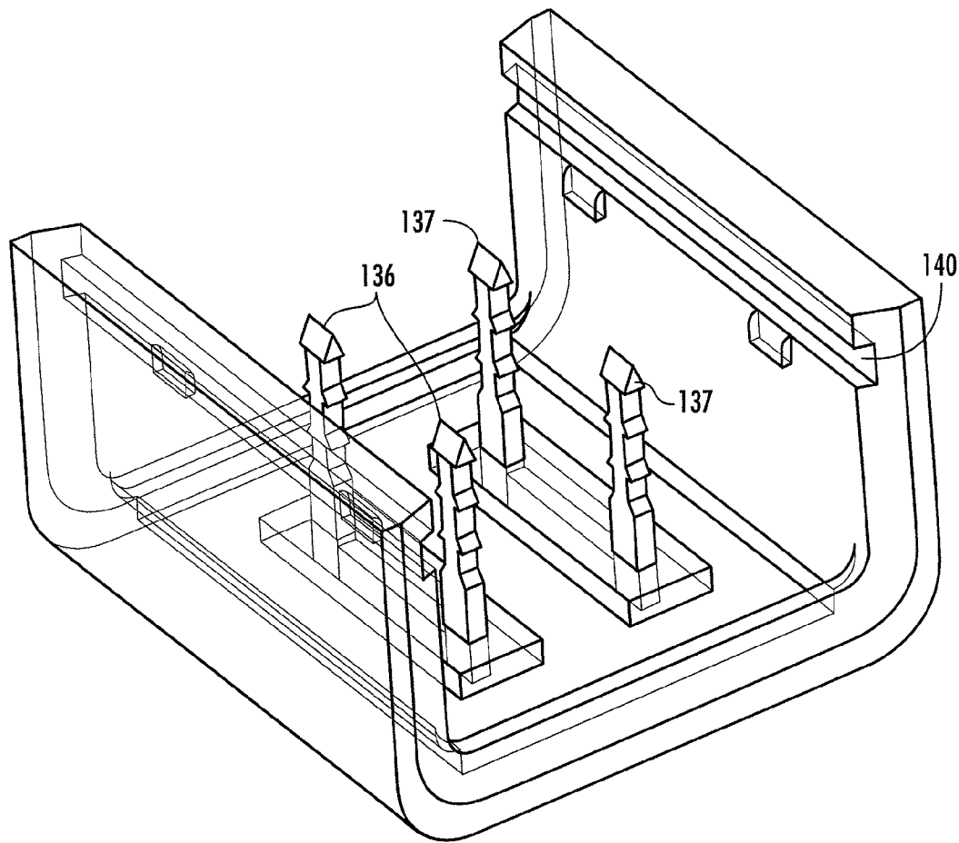
FIG. 26
