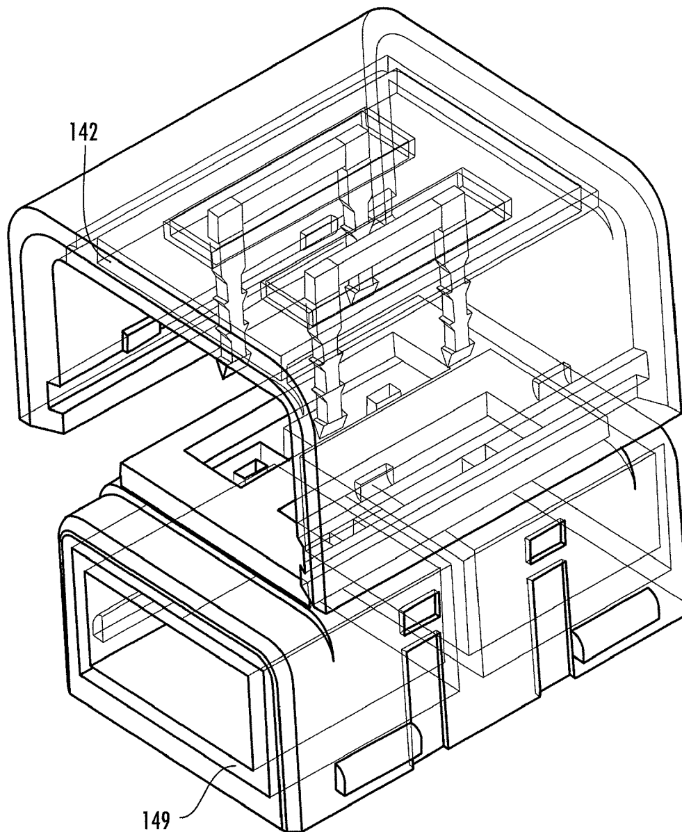
FIG. 24B
