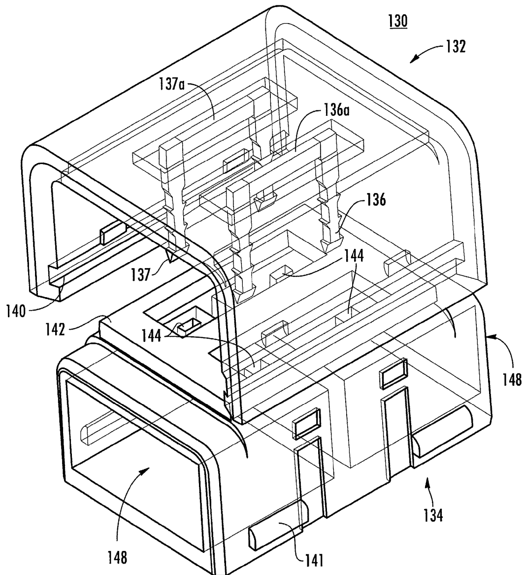
FIG. 24A
