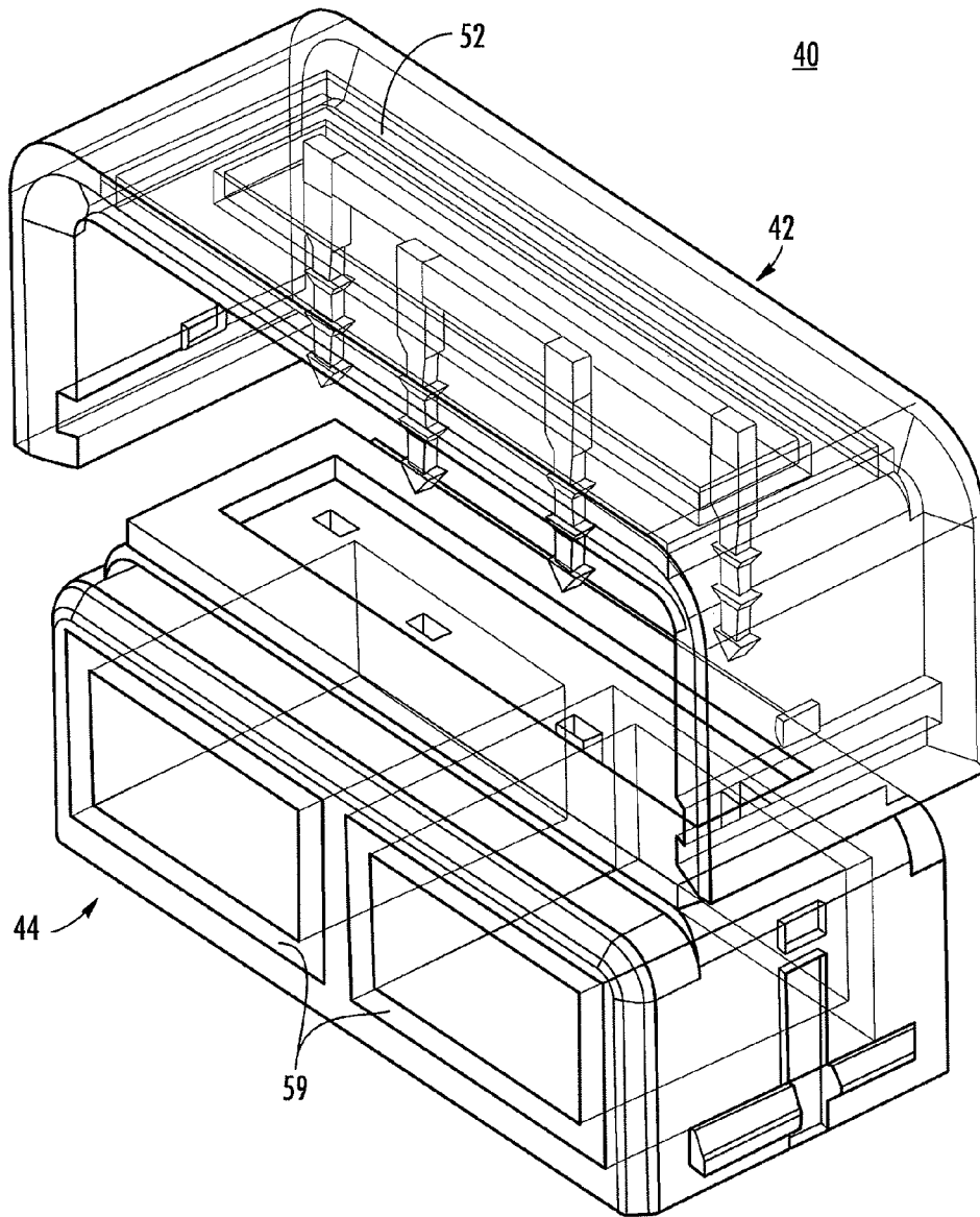
FIG. 11B
