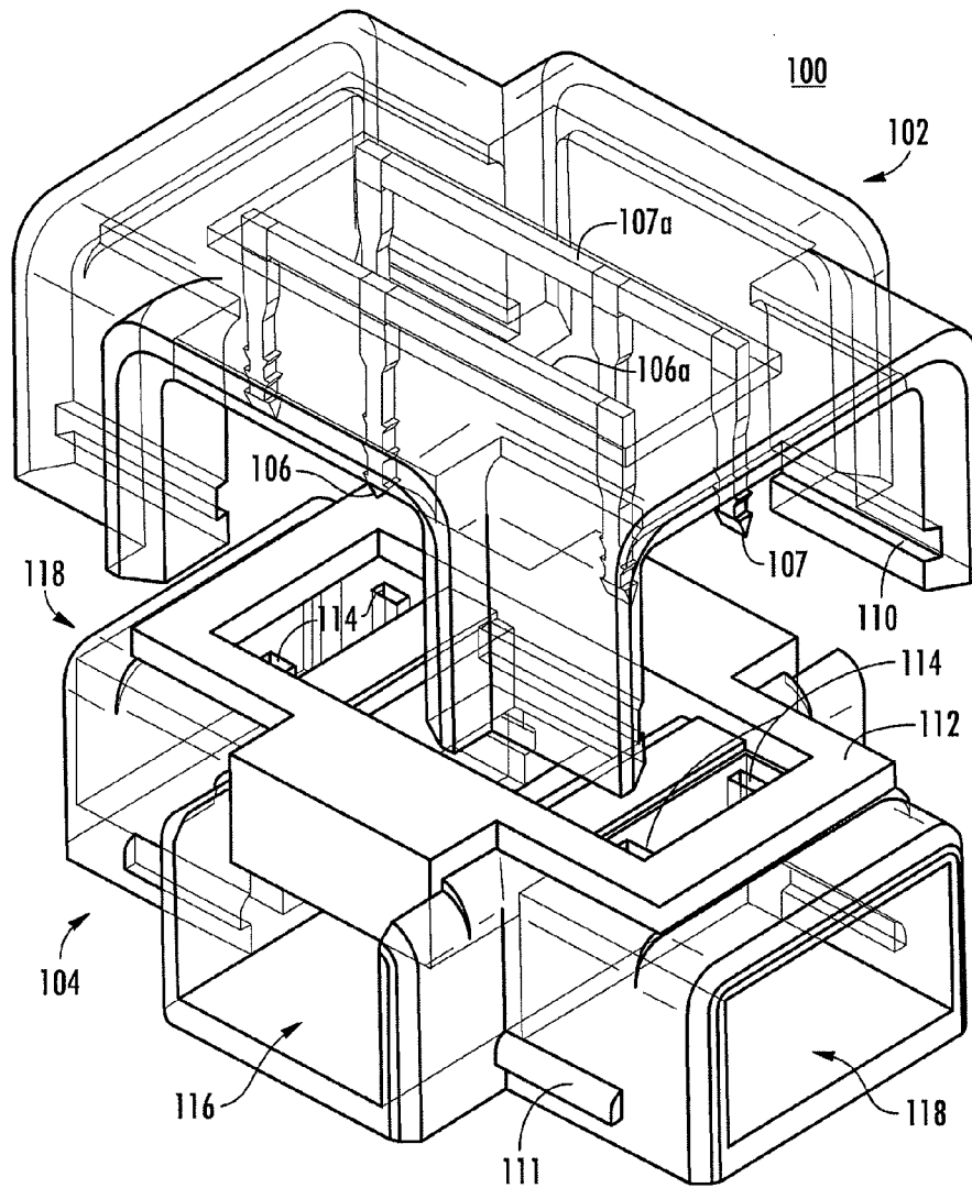
FIG. 19A
