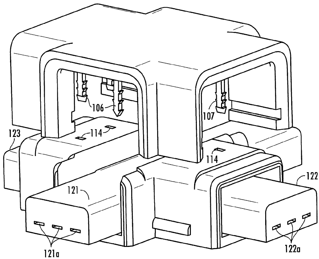
FIG. 22A
