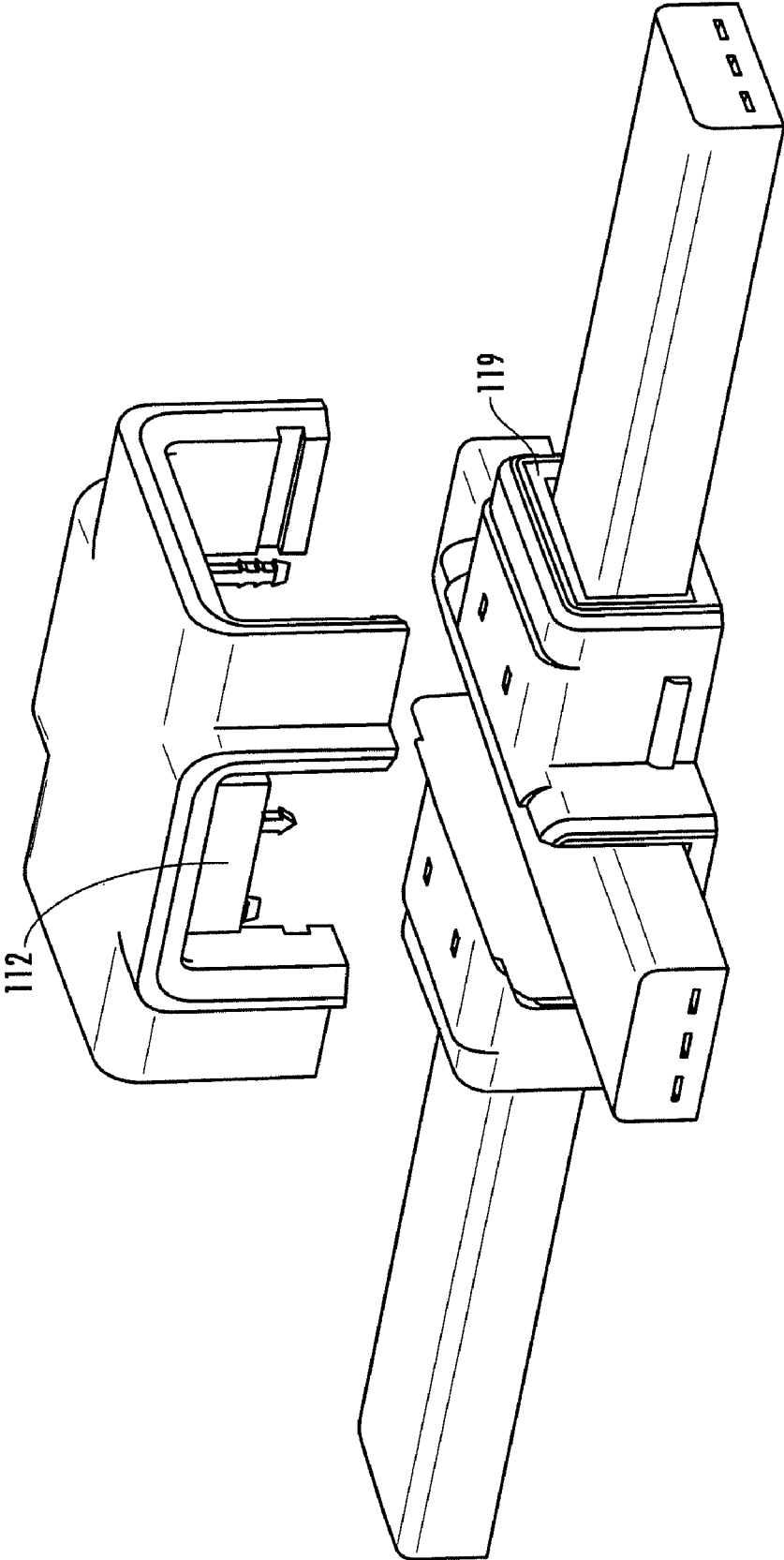
FIG. 22B
