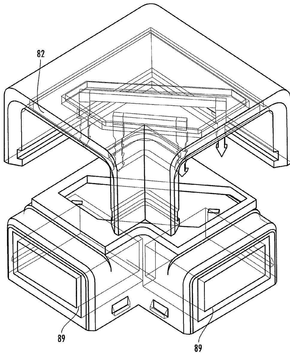
FIG. 14B
