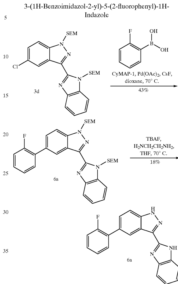
(a) Intermediate 6a—5-(2-Fluorophenyl)-1-[2-(trimethylsilyl)ethoxymethyl]-3-{1-[2-(trimethylsilyl)ethoxymethyl]-1H-benzoimidazol-2-yl]-1H-indazole:
