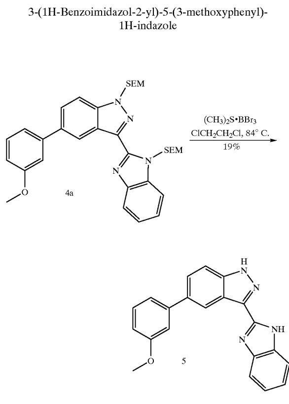
(a) Example 5—3-(1H-Benzoimidazol-2-yl)-5-(3-methoxyphenyl)-1H-indazole:
