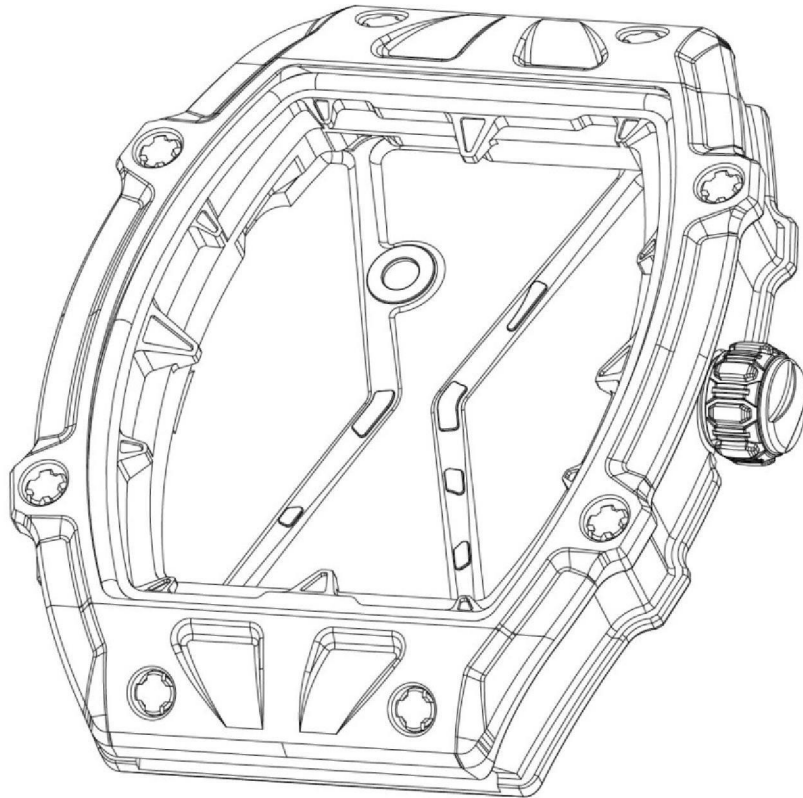
【立體圖1】
