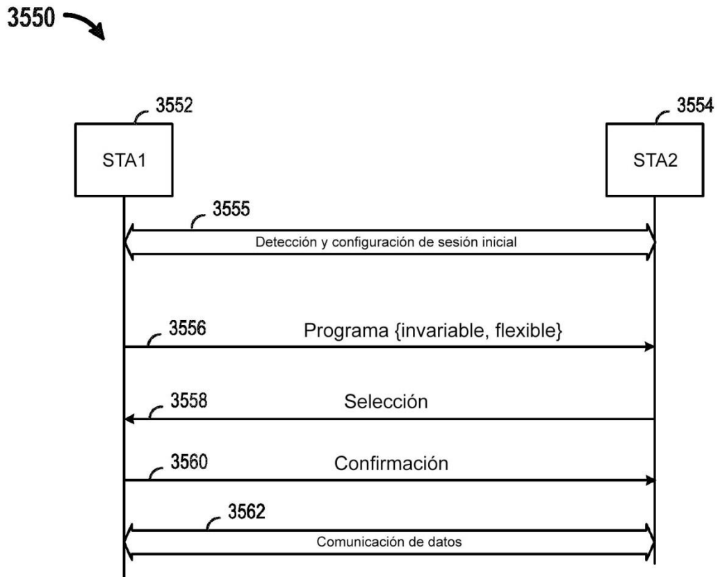
FIG. 35B
