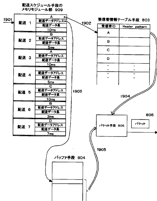
配送手段内の動作を説明する図
