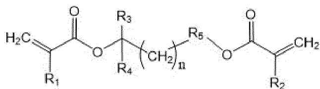
[Chemische Formel 1]
