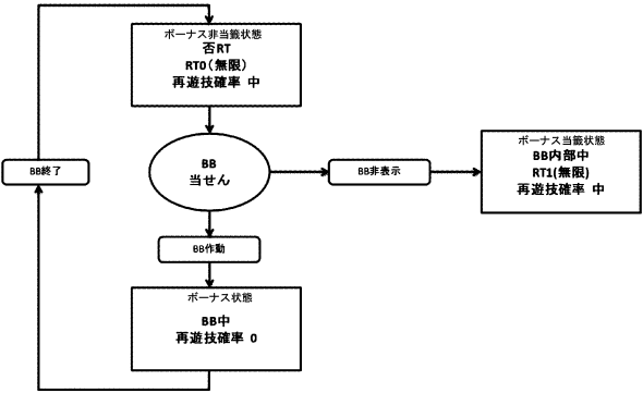
RT状態遷移図
