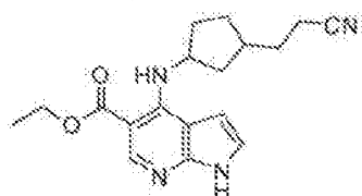
Cis
