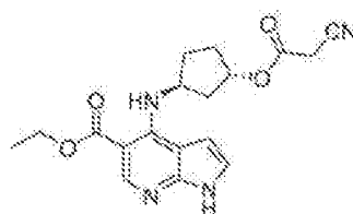
Trans enantiomer-1
