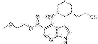
Cis - enantiomer 2
