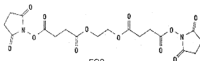
EGS M.W. 456.36 Spacer Arm 16.1 Å
