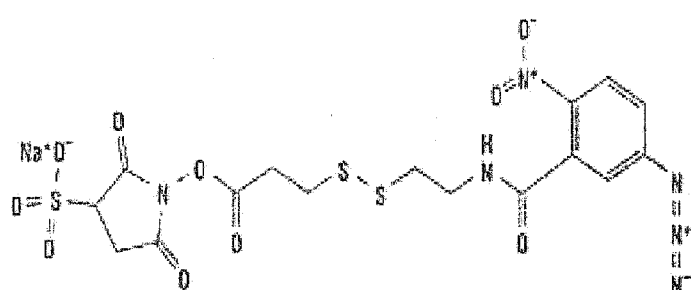
Sulfo-SAND M.W. 570.51 Spacer Arm 18.5 Å
