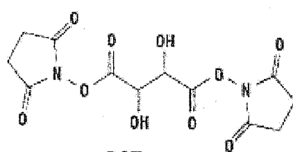
DST M.W. 344.24 Spacer Arm 6.4 Å
