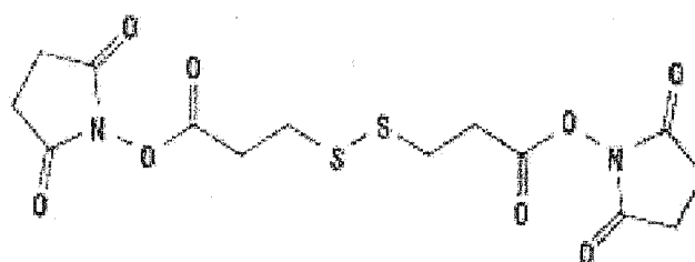
DSP M.W. 404.42 Spacer Arm 12.0 Å
