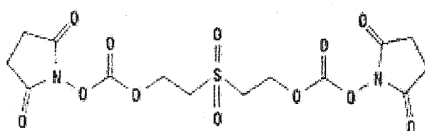
BSOCOES M.W. 436.35 Spacer Arm 13.0 Å
