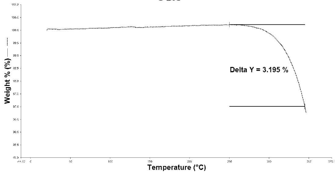
FIG. 6 TGA
