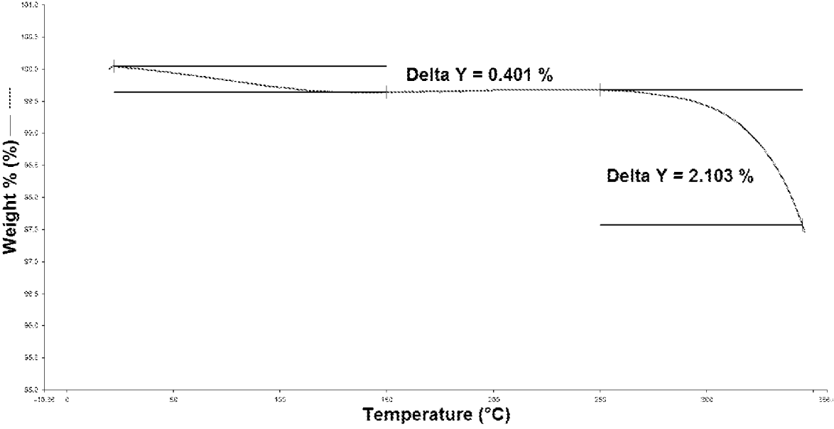
FIG. 3 TGA
