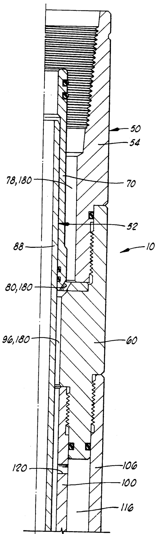
FIG. 5A
