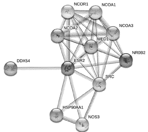
Estrogen Receptor 2 (ESR2)
