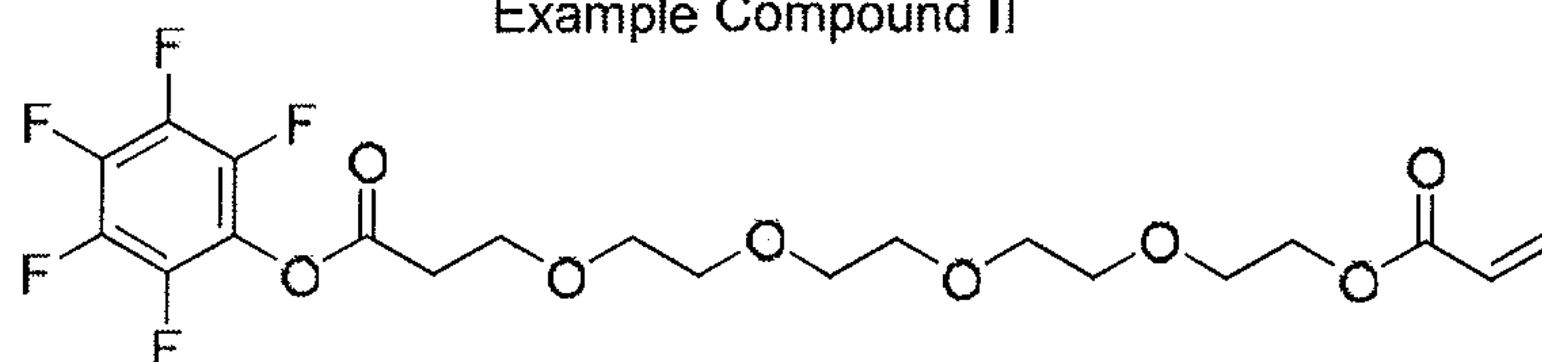
PFP-PEG5-Acrylate
