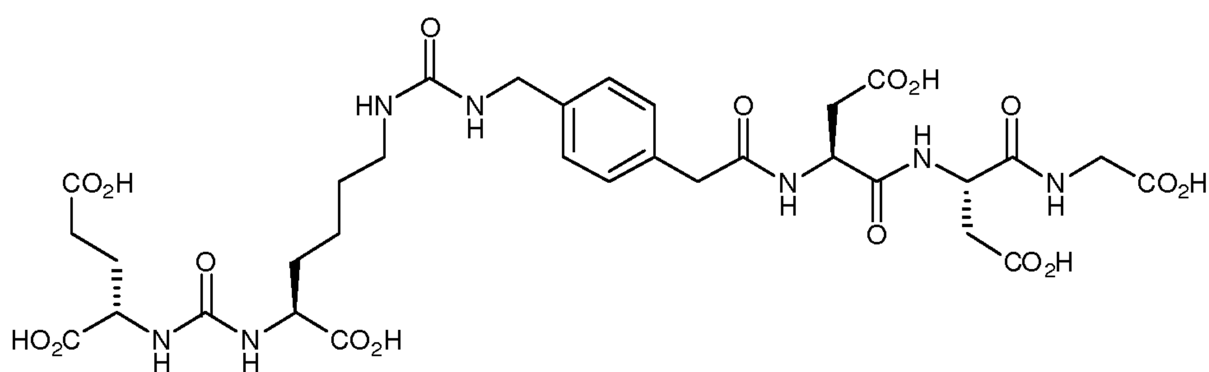
EC1168 (Exact Mass: 797.27 ; Mol. Wt.: 797.72)
