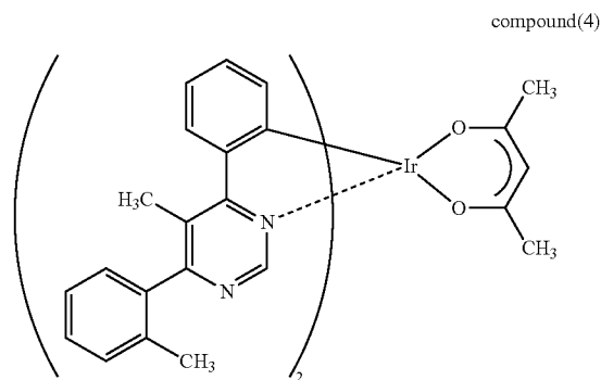
(xii) Ir(mpmpm) 2 (acac)
