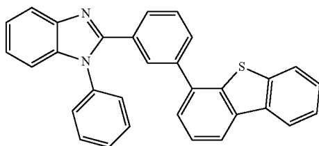
mDBTIm-II
