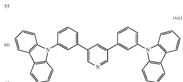
3,5DCzPPy
