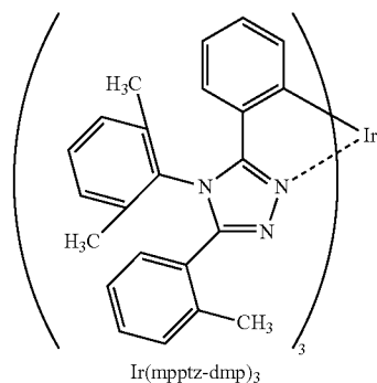
Ir(mpptz-dmp) 3
