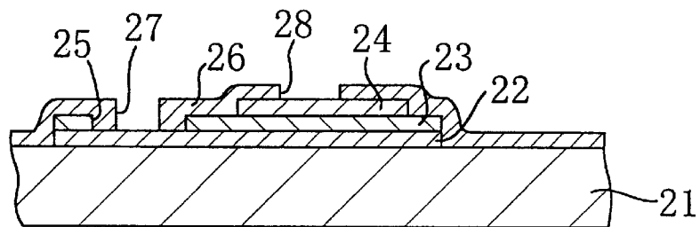
Fig. 10(d) PRIOR ART
