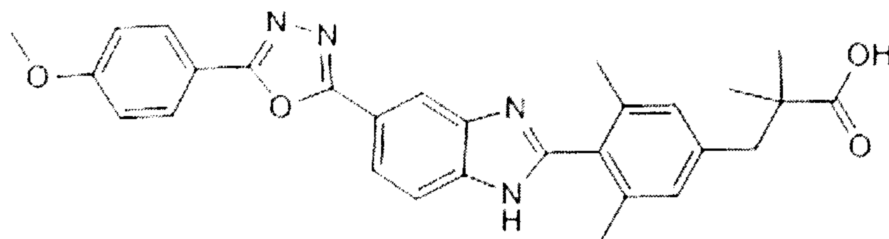
3-(4-(5-(5-(4-methoxyphenyl)-1,3,4-oxadiazol-2-yl)-1H-benzo[d]imidazol-2-yl)-3,5-dimethylphenyl)-2,2-dimethylpropanoic acid
